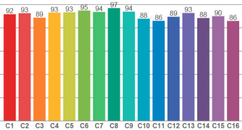
TM30: 91.2
